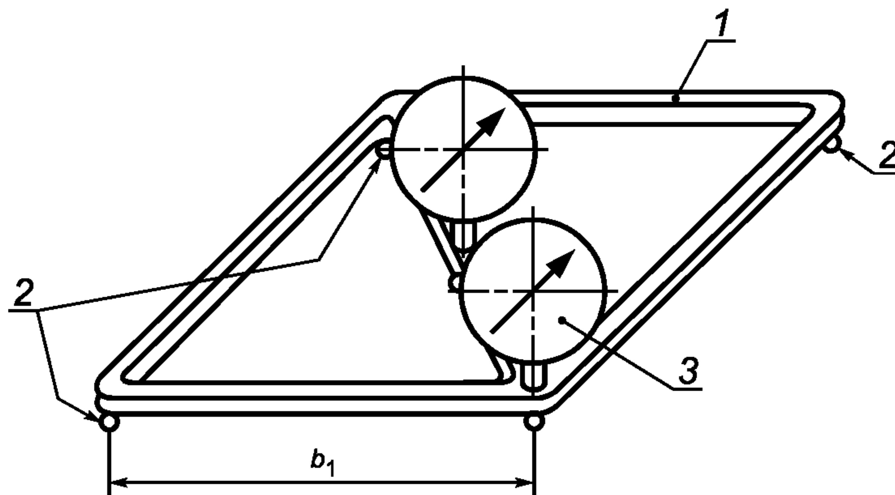
Схема прибора для измерения отклонений от плоскостности
